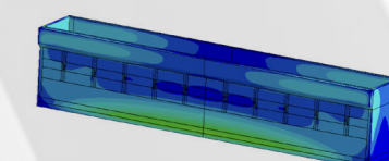
Максимальные сжимающие напряжения наблюдаются в области опоры и равны 8,0603 МПа
